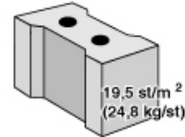
BIA 32-24 klinker LxBxH = 200 x 320 x 240 (47,5 ltr specie per m 2 )
