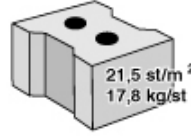
BIA 26-19 klinker LxBxH = 250x265x190 (40,5 ltr specie per m 2 )
