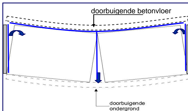
Gevulde dilatatievoegen, aan boven- en zijkanten vullen met Flexschuim ®
